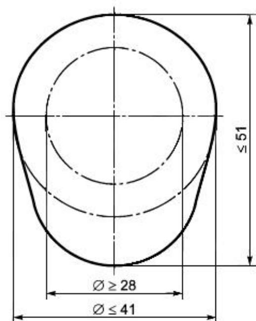
Рисунок 8 - Размеры поперечного сечения перекладин оборудования для лазания
