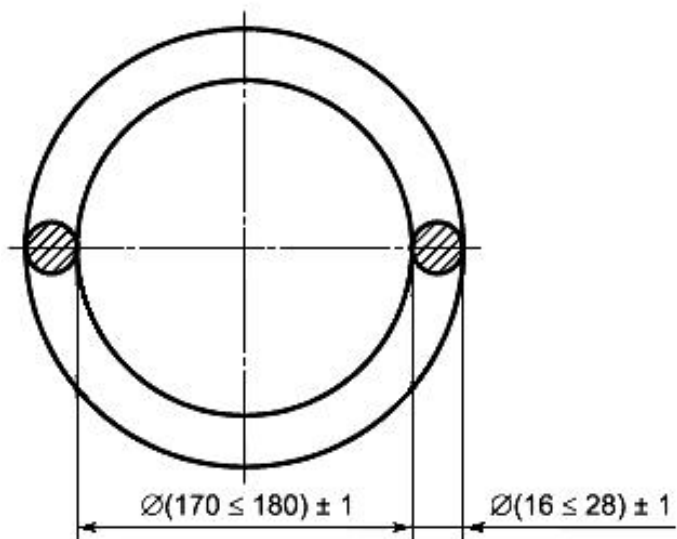
Рисунок 5 - Размеры кольца
